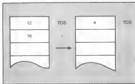
Bild 2. So verändert sich der Stack bei der Subtraktion
